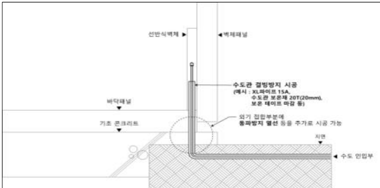
[수도관 결빙방지 시공 개략도]
